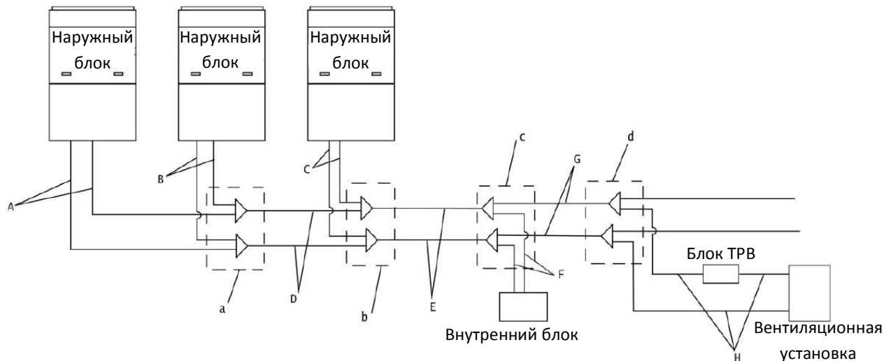
Рис. 3.5.1: Подключение одного комплекта АНУ-KIT к одной вентиляционной установке
