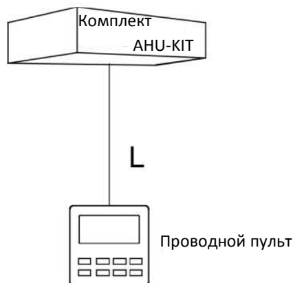
Рис. 3.3.1: Подключение одного проводного пульта к одному комплекту АНУ-КИТ.
