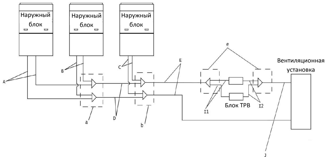
Рис. 3.5.2: Подключение нескольких комплектов АНУ-KIT к одной вентиляционной установке
