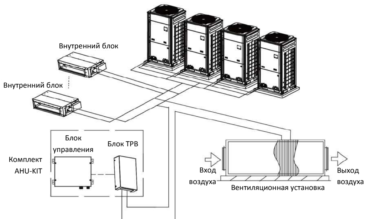
Рис.2.5.3: Подключение комплекта АНУ-kit к наружному блоку совместно с обычными внутренними блоками
