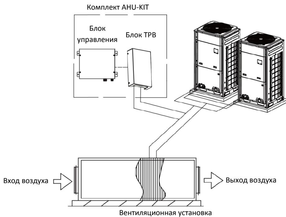
Рис. 2.5.2: Подключение комплекта АНУ-КІТ к модульному наружному блоку
