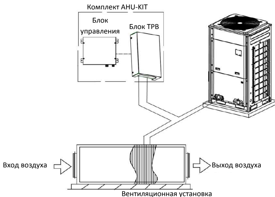
Рис. 2.5.1: Подключение комплекта АНУ-КІТ к отдельному наружному блоку
