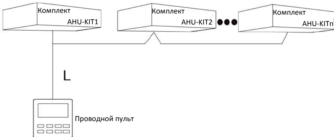
Рис. 3.3.2: Подключение одного проводного пульта к нескольким комплектам АНУ-КИТ.
